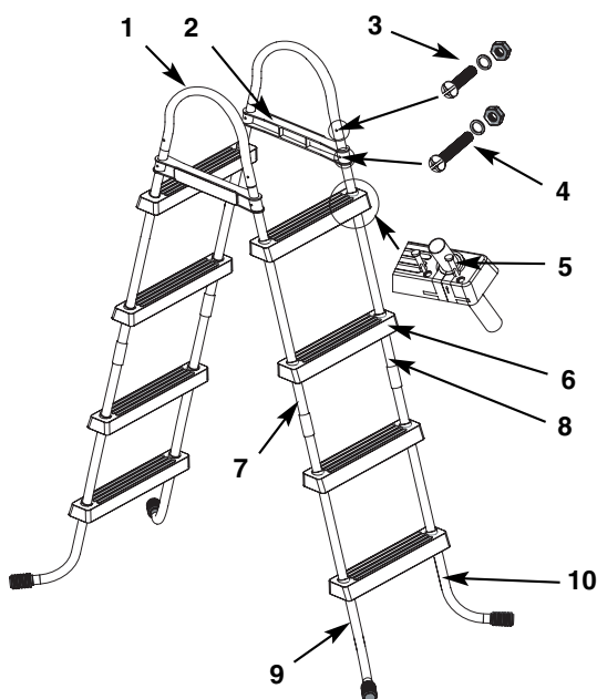
Leiter 48" (122 cm) Modell
