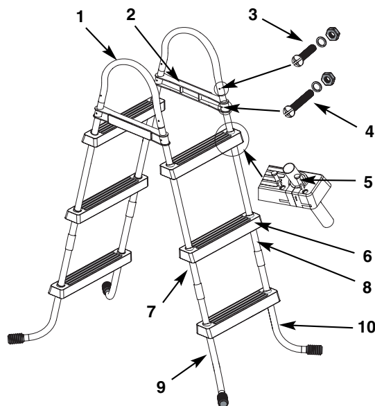
Leiter 36" (91cm) & 42" (107cm) Modelle
